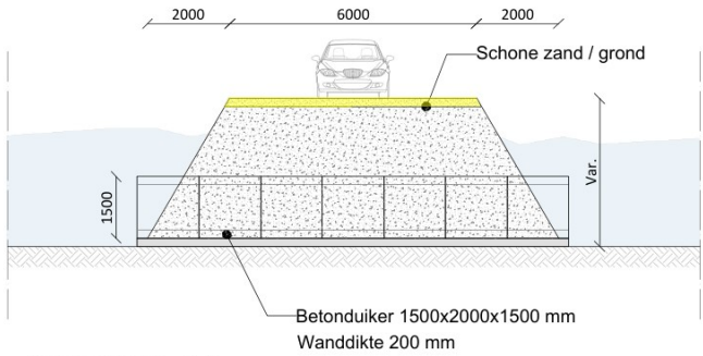
Doorsnede A-A Schaal: 1:200
